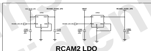
RCAM2 LDO
