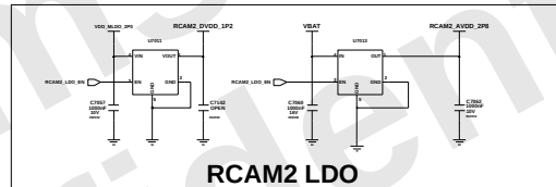
RCAM2 LDO
